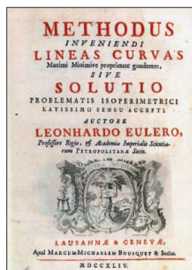
«Метод нахождения кривых линий...» Трактат Леонарда Эйлера, 1744 г.
