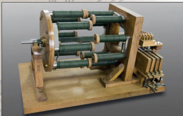
Электродвигатель Б. С. Якоби.
