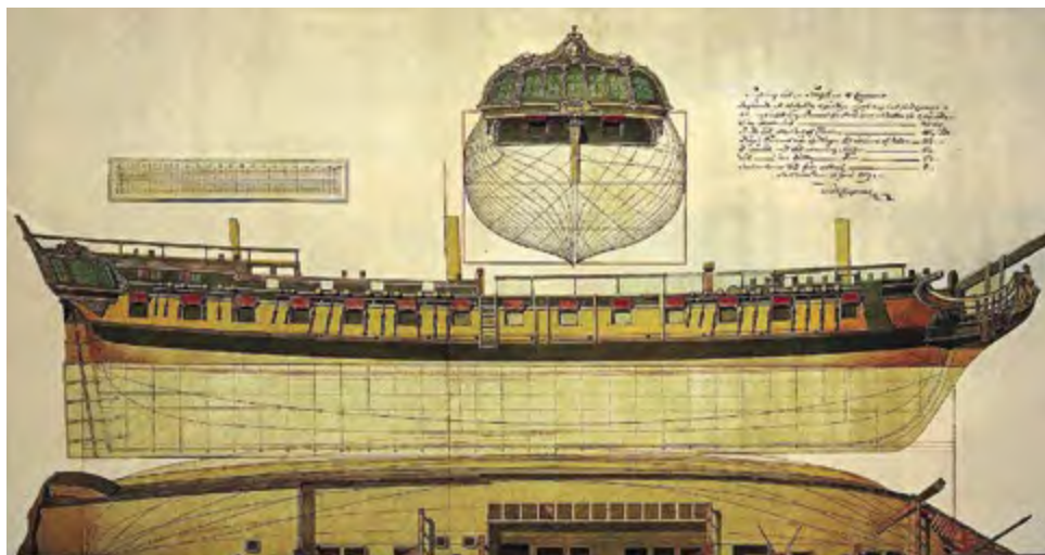
Теоретический чертеж фрегата «Венус». 1783 год
